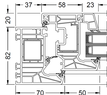
Schüco Living 82 MD
