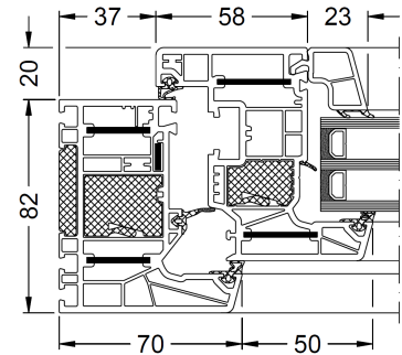
Schüco Living Alu Inside
